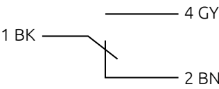
1 A 230 V AC – 250 V DC 40 W Schaltplan
