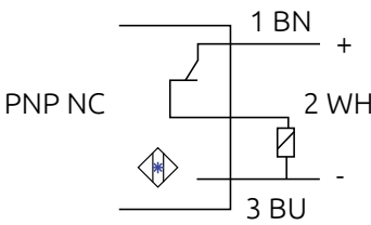
Schaltplan
